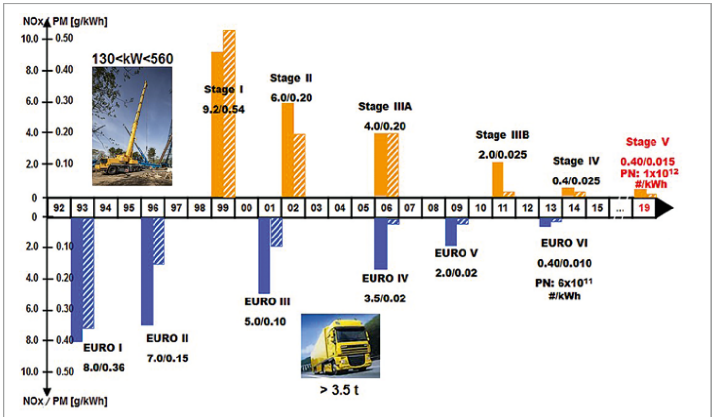
Übersicht Abgasstufenentwicklung.
