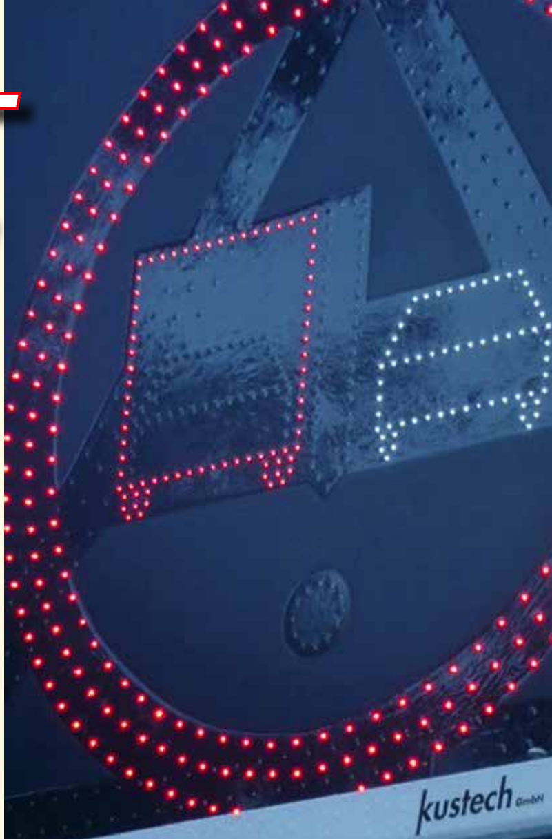
Immer noch gut zu erkennen: So sieht es aus, wenn der Abstrahlwinkel mehr als 70 Grad beträgt.
